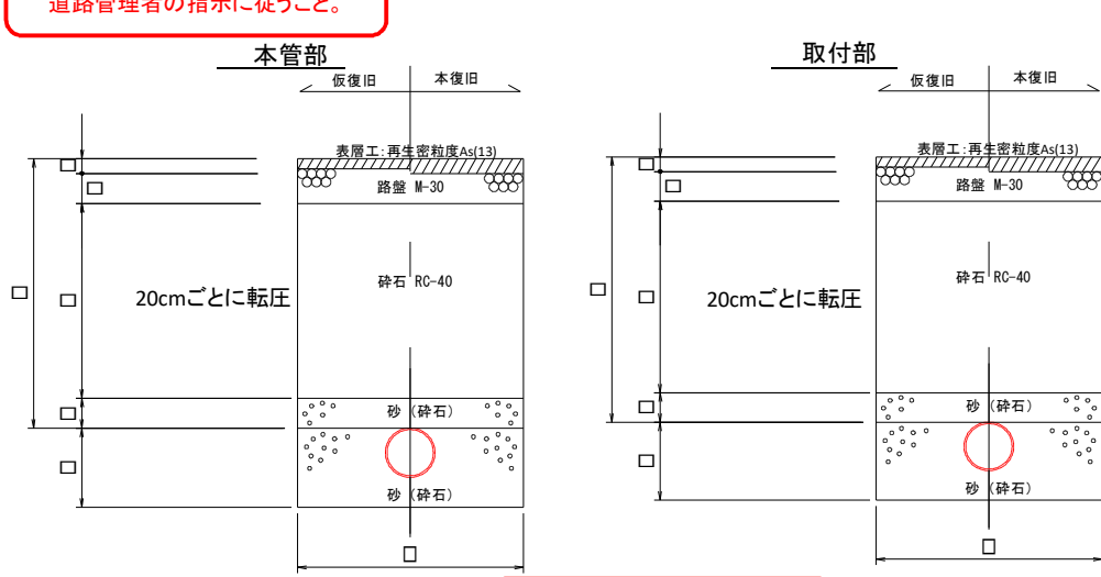
掘削断面図 S=1/100
