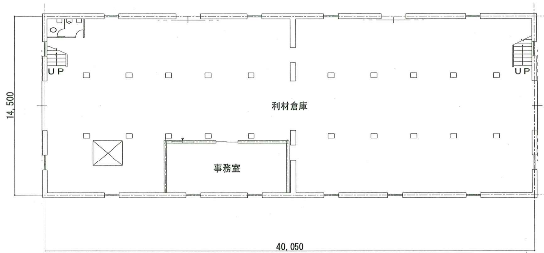
倉庫 1 階平面図 S=1/300
