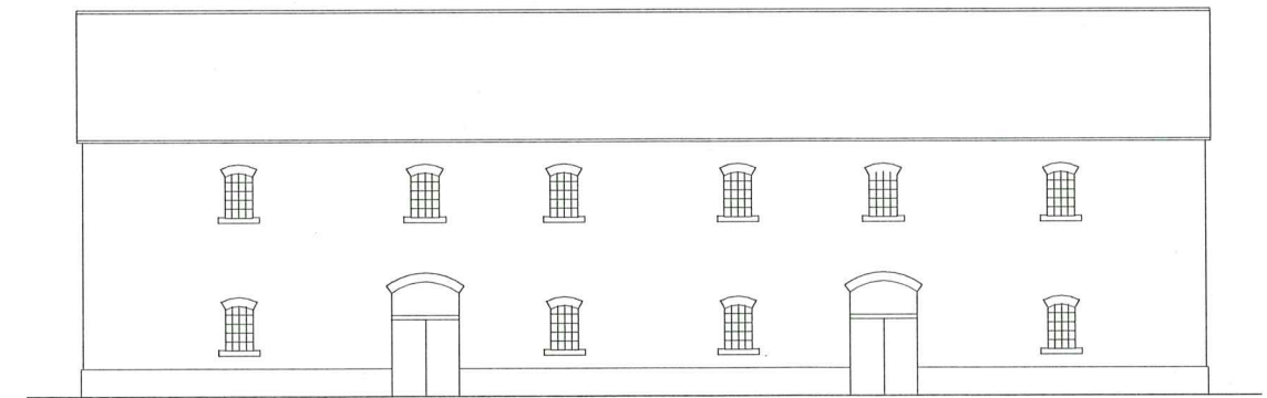
北側立面
