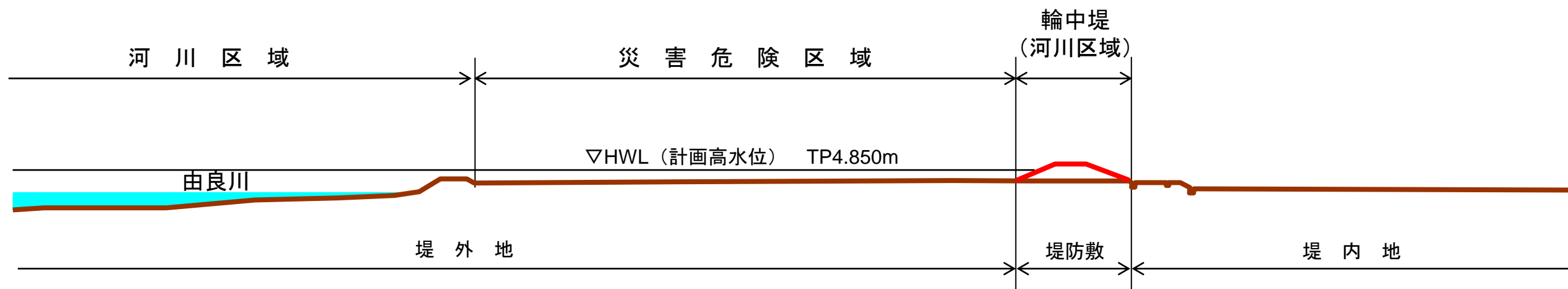
横断図 (4.4km付近) a-a'
