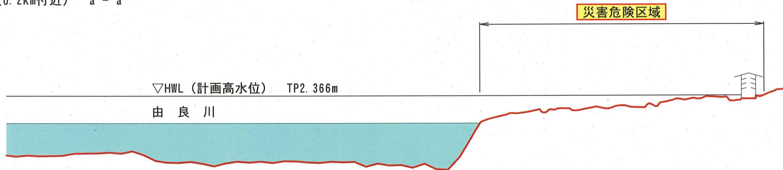
横断図 (0.2km付近) a - a'
