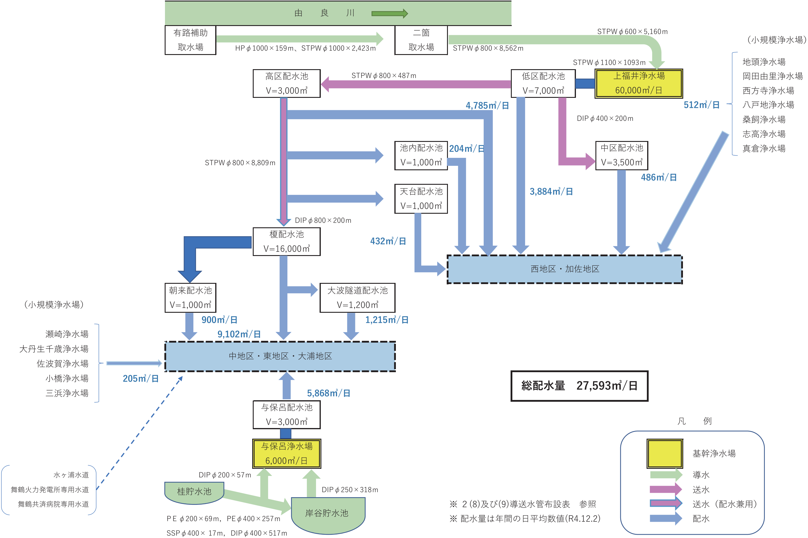
(6) 配水量分布図
