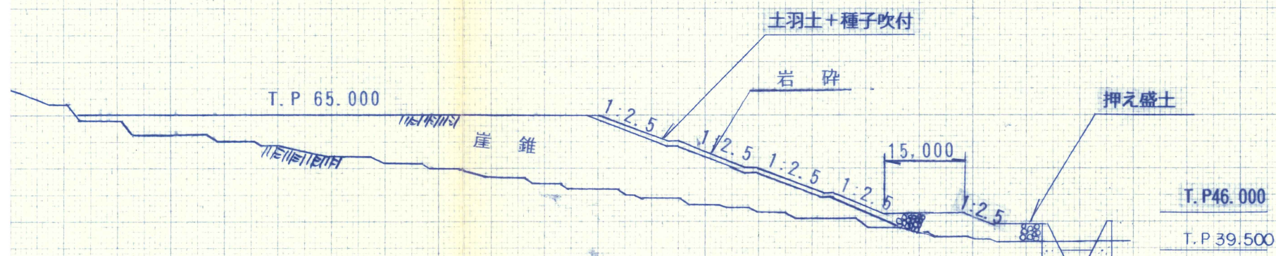
① — ① 断面図
