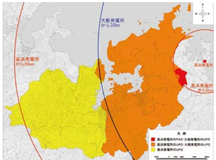
高浜発電所のPAZ・UPZと大飯発電所のUPZ
