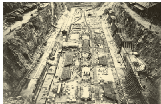
▲3号ドック(ジャパンマリンユナイテッド株式会社舞鶴営業所提供)
