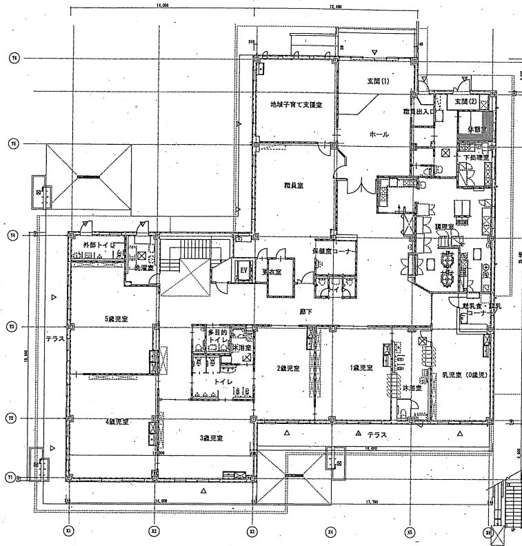
1階平面図
