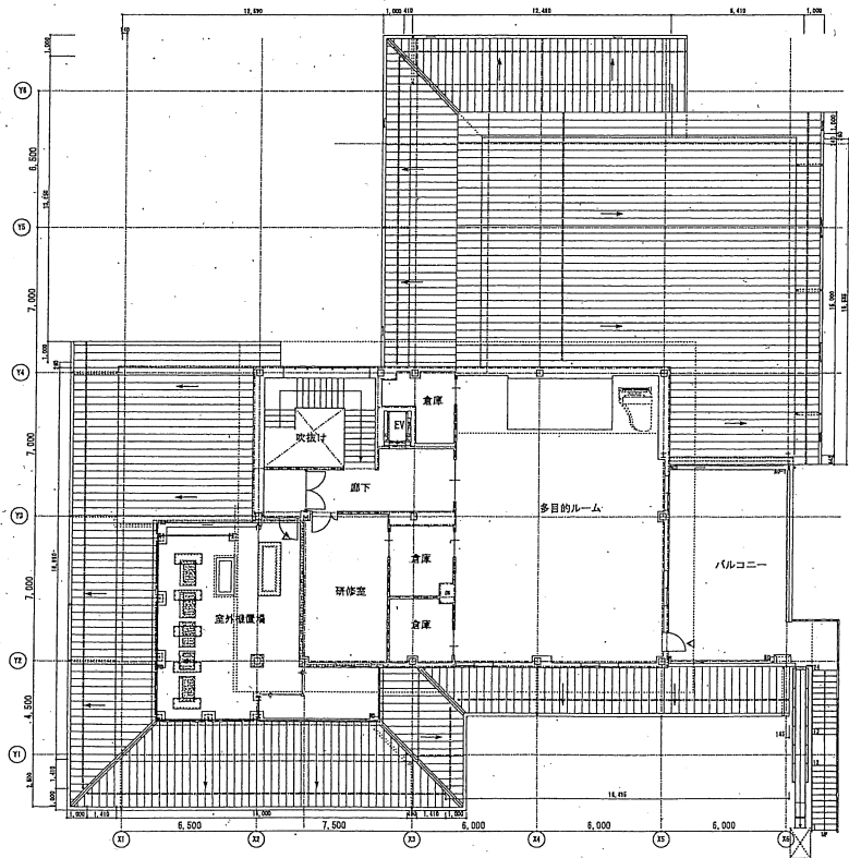
2階平面図
