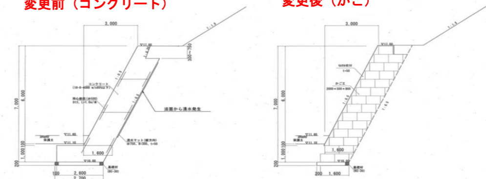
変更後（かご）
