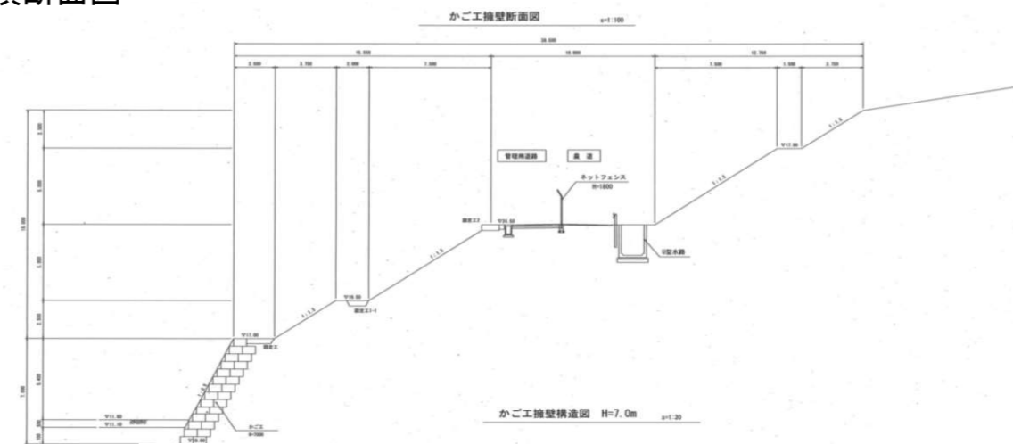
変更後（かご）
