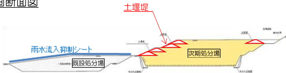
埋立計画断面図
